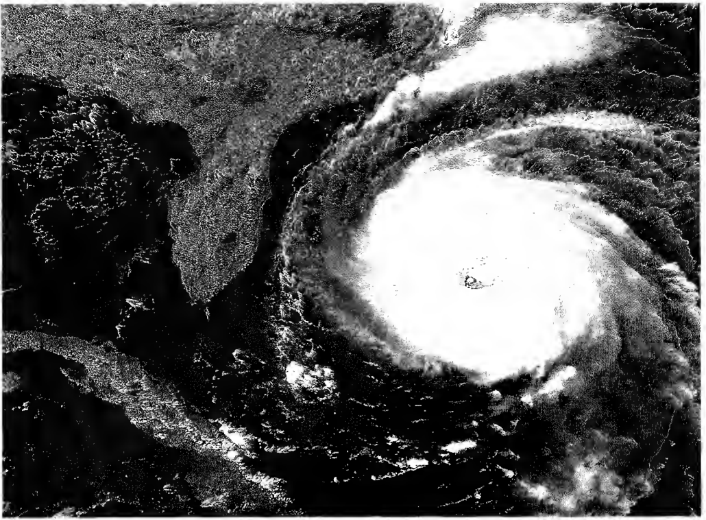
العواصف والرياح تتكون في نطيق الرجع Troposphere
